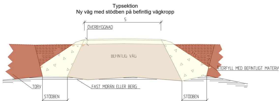
FIGUR 14. EXEMPEL PÅ TYPSEKTION FÖR NY VÄG MED STÖDBEN PÅ BEFINTLIG VÄGGROPP (KÄLLA: ARCTAN AB)
